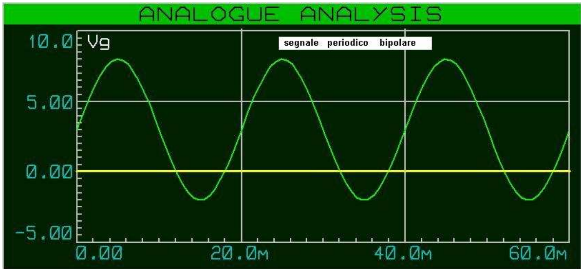
(SINUSOIDE CON OFFSET)
